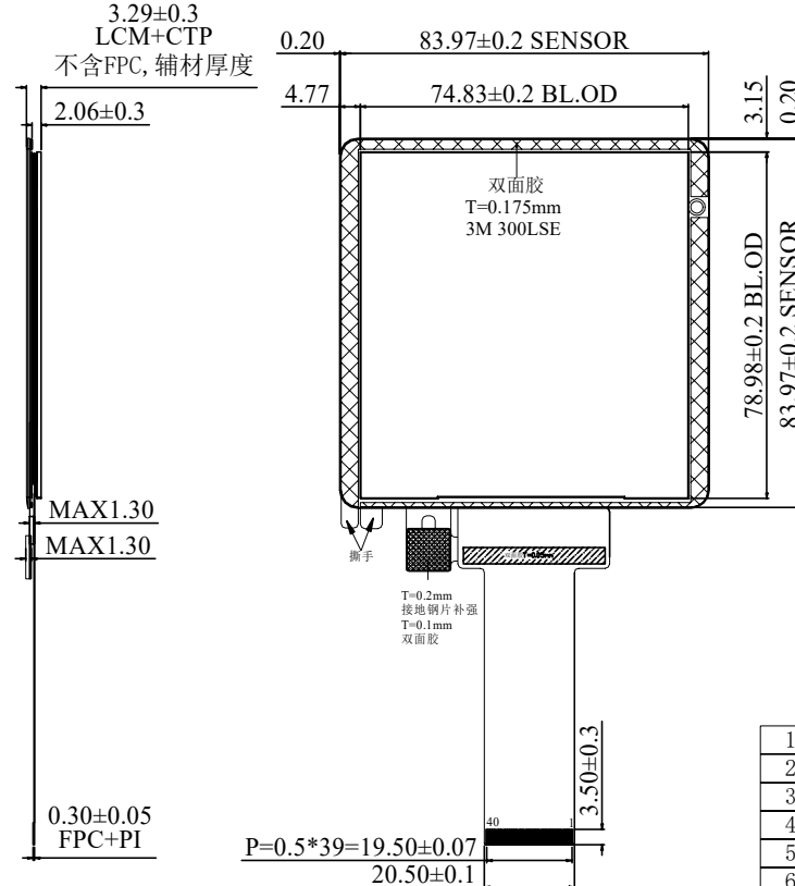
侧视图
